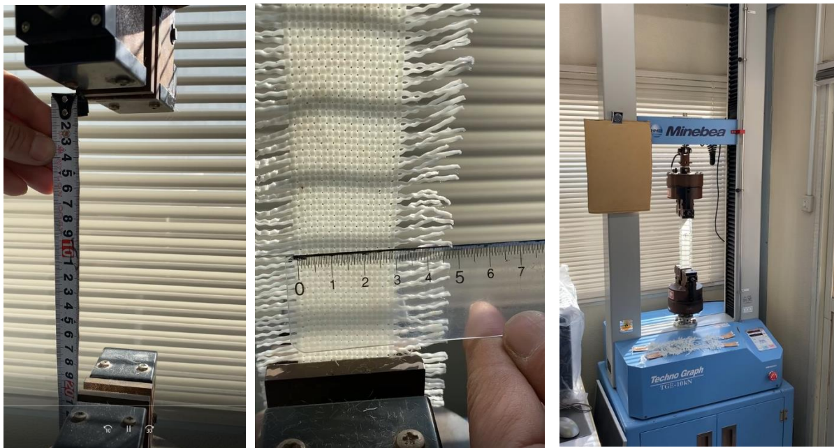
カーテン残存強度確認 引張試験状況
