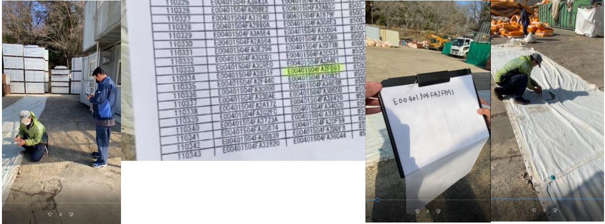
カーテン残存強度確認 試験体採取状況
