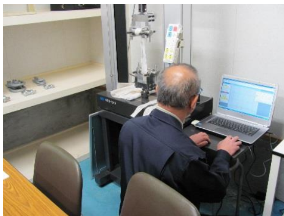
引張試験状況
